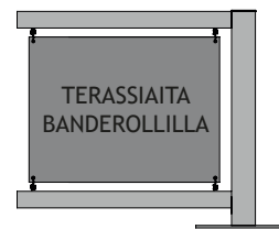
Jatkomodduuli 1000 x 900 mm Moduulin osat: jalka, muovikansi ja bänderolli
